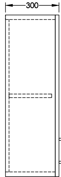
END ELEVATION
